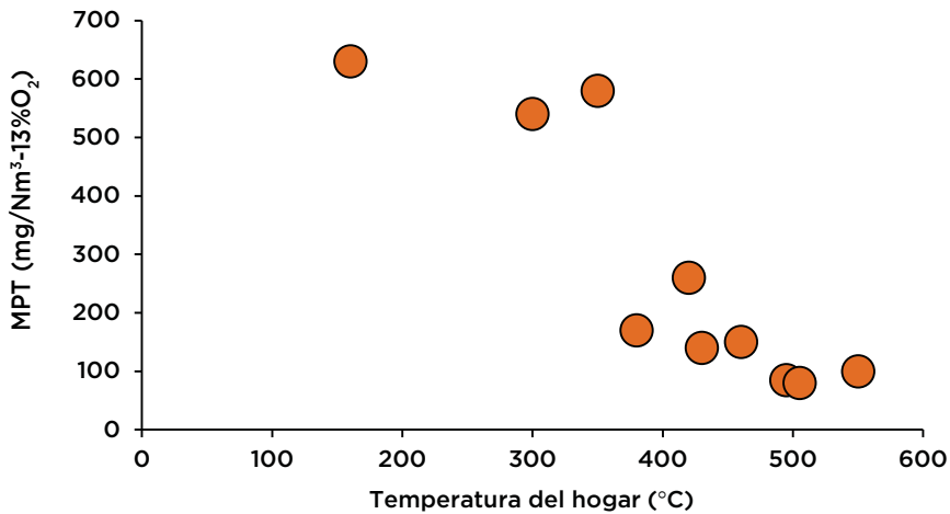
Figura 11 Emisión total de material particulado (MPT) en función de la temperatura del hogar
