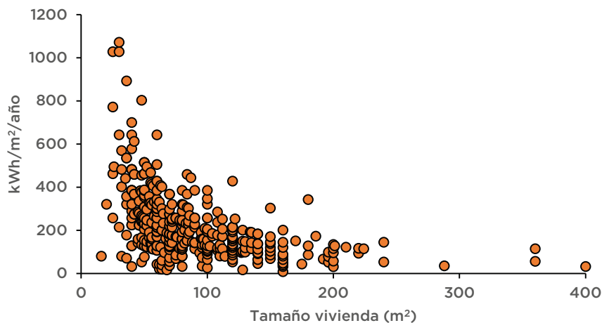
Figura 6. Consumo de energía para calefacción de acuerdo al tamaño de la vivienda
